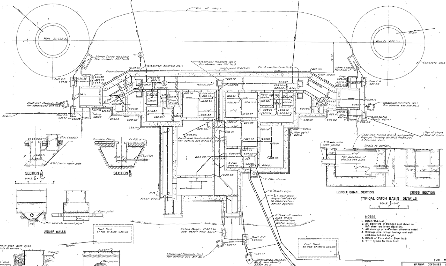
DRAINAGE LAYOUT SCALE: 1/8" = 1'-0"
